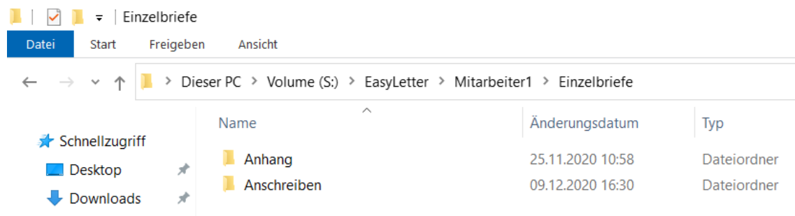
Abbildung 1.5: Aufbau Einzelbriefe
