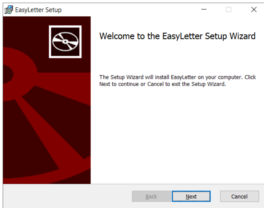
Abbildung 2.4: EasyLetterSetup.msi Willkommen
