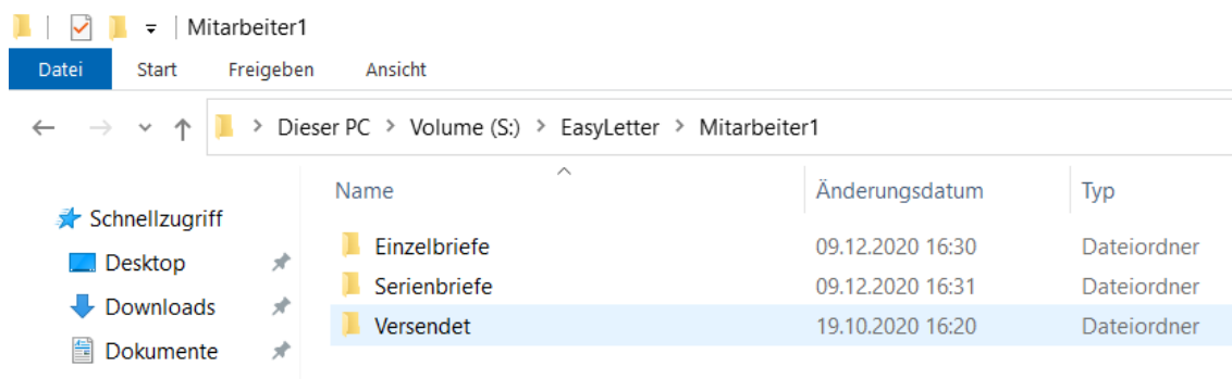
Abbildung 1.3: Aufbau Auftragsverzeichniss
