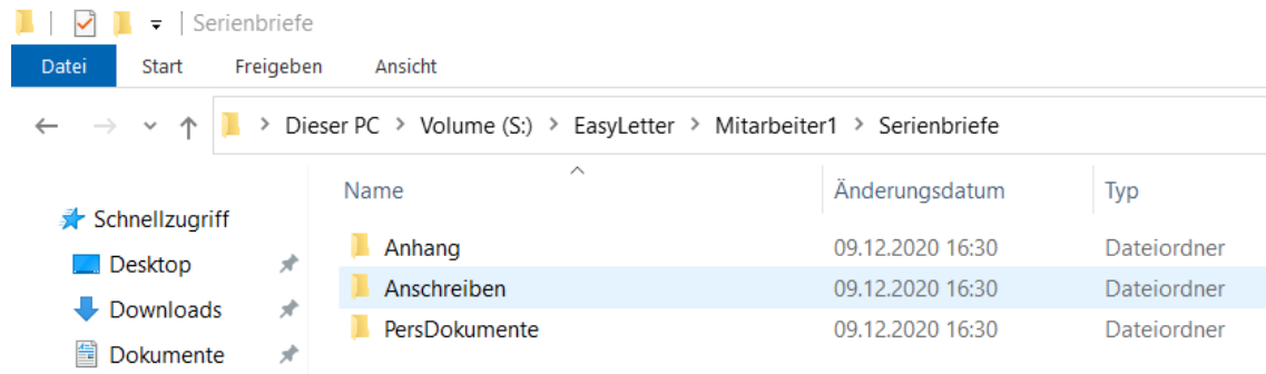
Abbildung 1.4: Aufbau Serienbriefe
