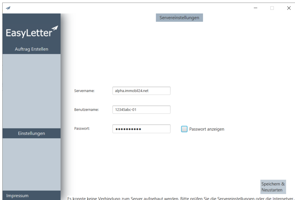
Abbildung 2.6: Konfiguration Server
